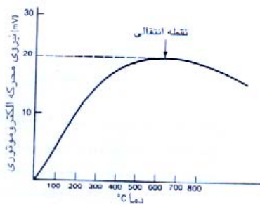
شکل ۸-۳ یک مشخصه ترموکوپل، نشاندهنده انحنا و نقطه انتقالی است که در آن مشخصه معکوس می‌شود. تعداد کمی از ترکیبات فلزی وجود دارند (مانند مس / نقره) که دارای نقطه انتقالی نیستند اما دارای خروجی ولتاژ بسیار ضعیفی هستند.
