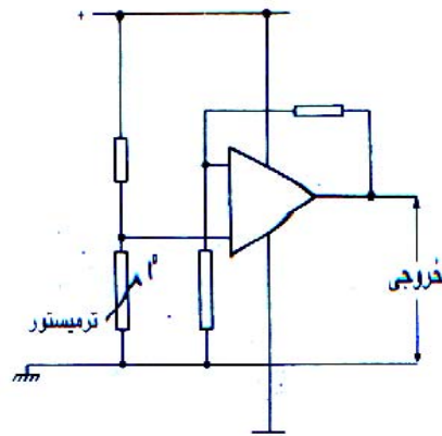
شکل ۴-۱۳ یک مدار تشخیص دهنده دما با استفاده از ترمیستور NTC که در آن از یک تقویت کننده عملیاتی استفاده شده است. حساسیت مدار را می توان با تغییر دادن نسبت فیدبک تقویت کننده، افزایش و یا کاهش داد.
