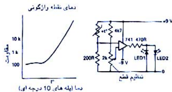
شکل ۱۴-۴ مشخصه یک ترمیستور PTC که جهت تشخیص اضافه دما به کار می رود.
